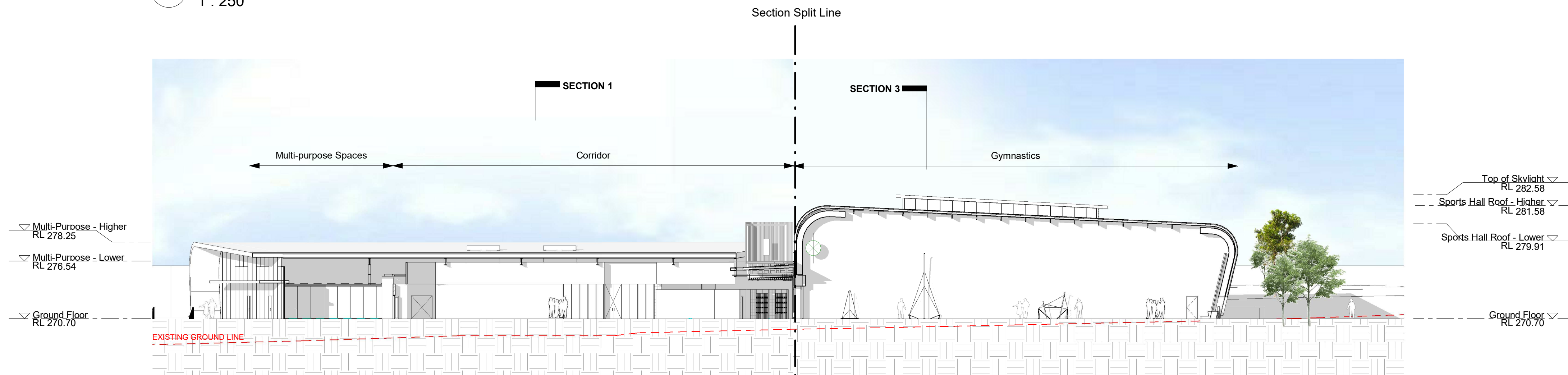
2 Section 2 1 : 250
