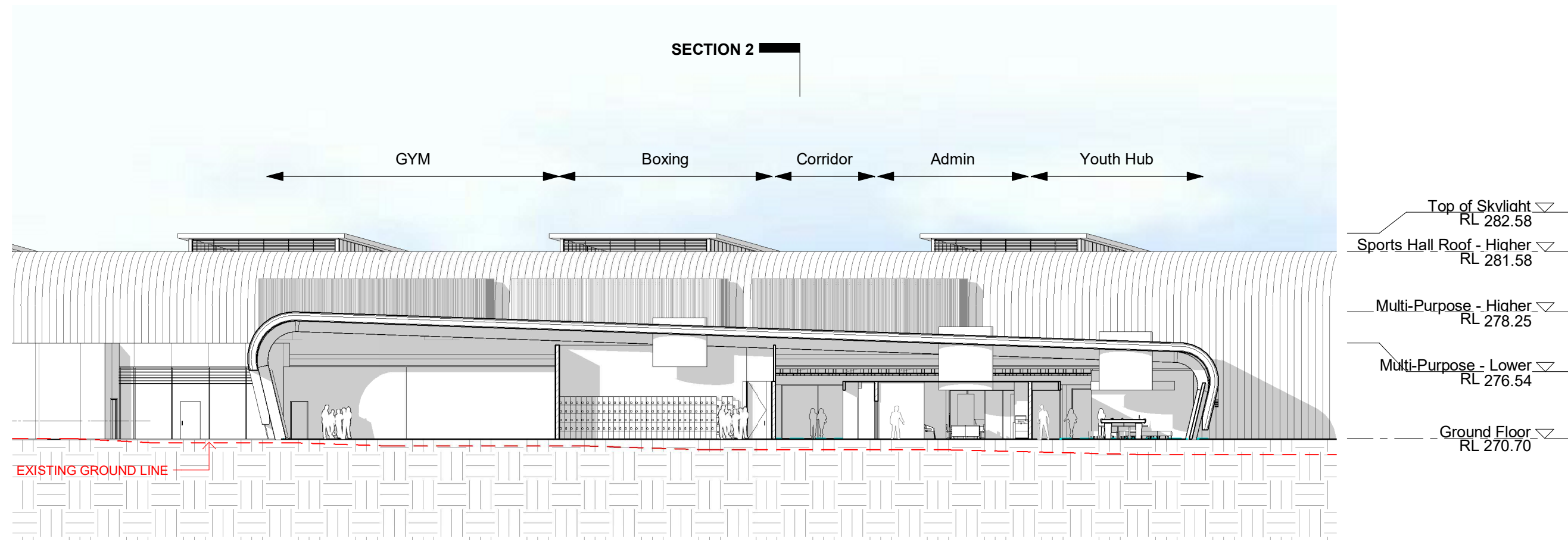
1 Section 1 1 : 250
